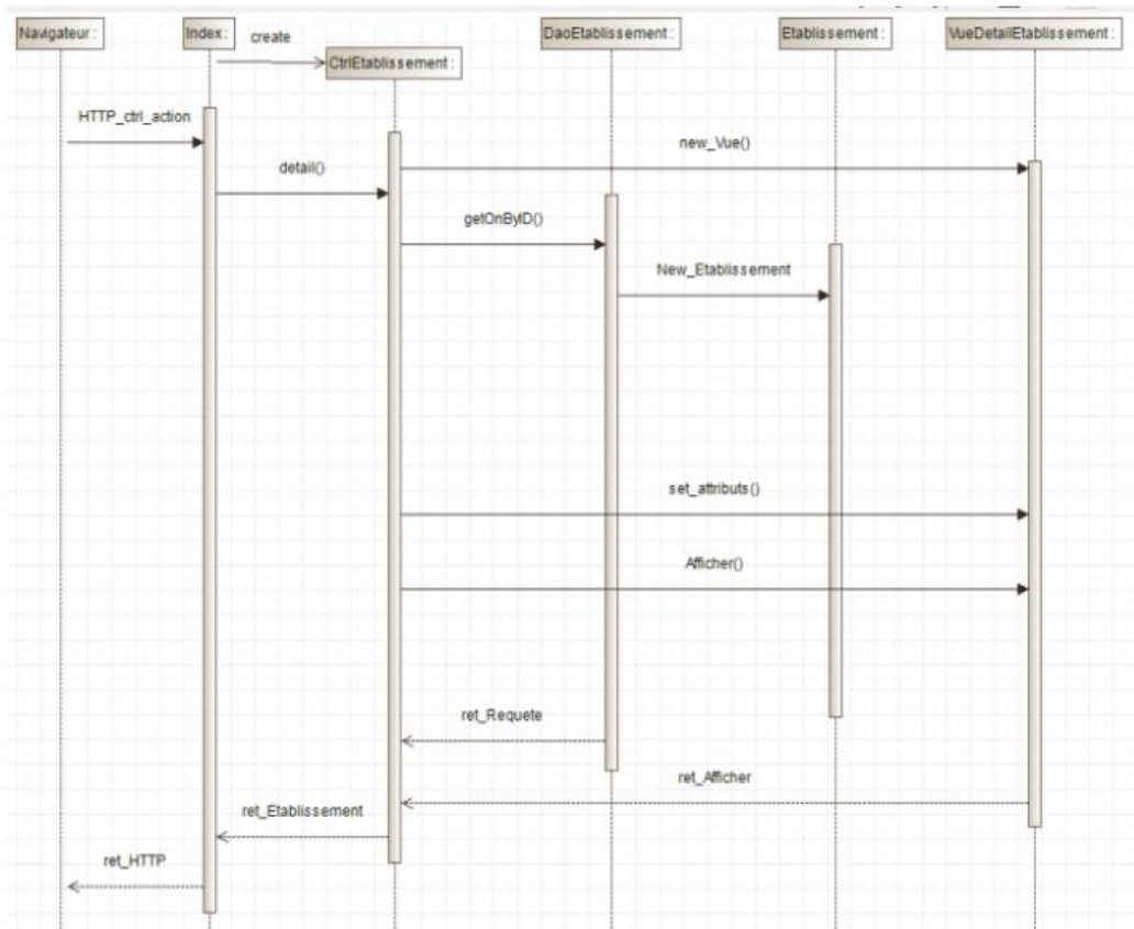
Figure 2 : Diagramme de séquence pour la modification
