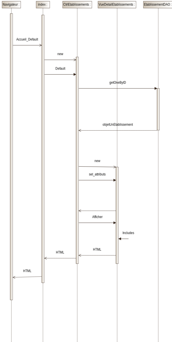
Figure 1 : Diagramme de séquence pour la consultation
